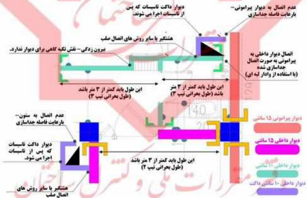
شکل پ-۱۱-۶ جزئیاتی در خصوص دیوارهای اطراف داکت تاسیسات و دیوارهای دارای بیرون زدگی
