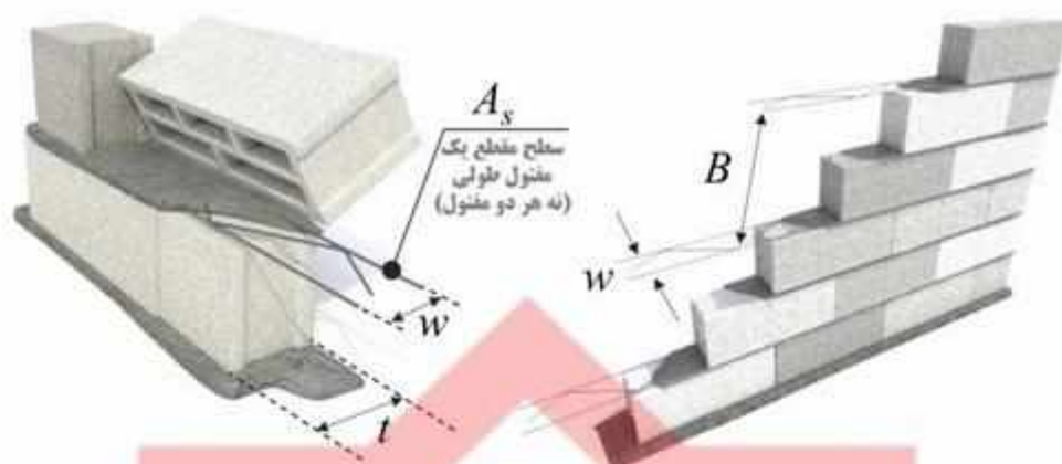
شکل ۲-۳ کمیت‌های مورد نیاز برای محاسبه ظرفیت خمشی افقی دیوارهای بتنی مسلح به میلگرد بستر.
