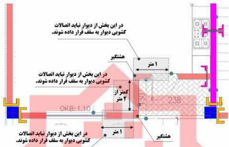
شکل پ-۶-۱۴ لزوم رعایت حداقل فاصله ۱ متری بین اتصالات کشویی دیوار به سقف از محل هشکگر
