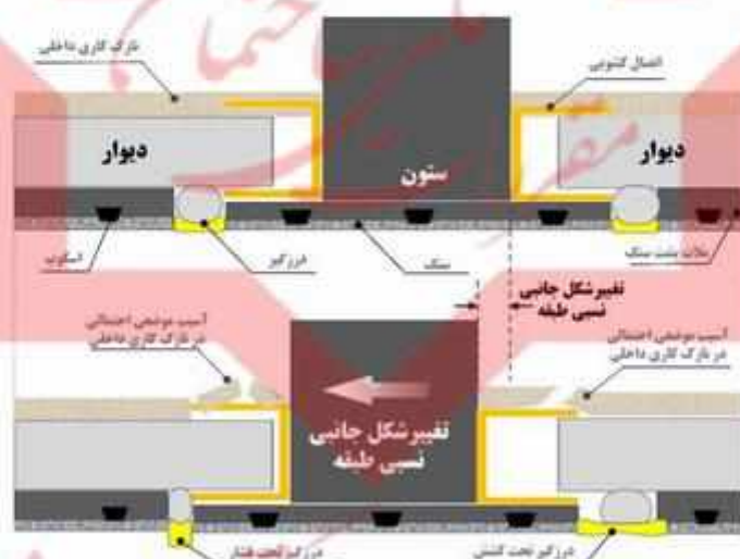
شکل ۴-۳۲ جداسازی نمای چسبیده شده از ستون با عبور نما از روی ستون
