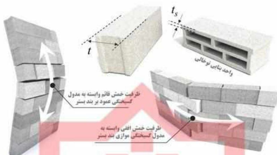
شکل ۳-۱ کمیت‌های مورد نیاز برای محاسبه ظرفیت خمشی قائم و افقی دیوارهای بنایی غیرمسلح.
