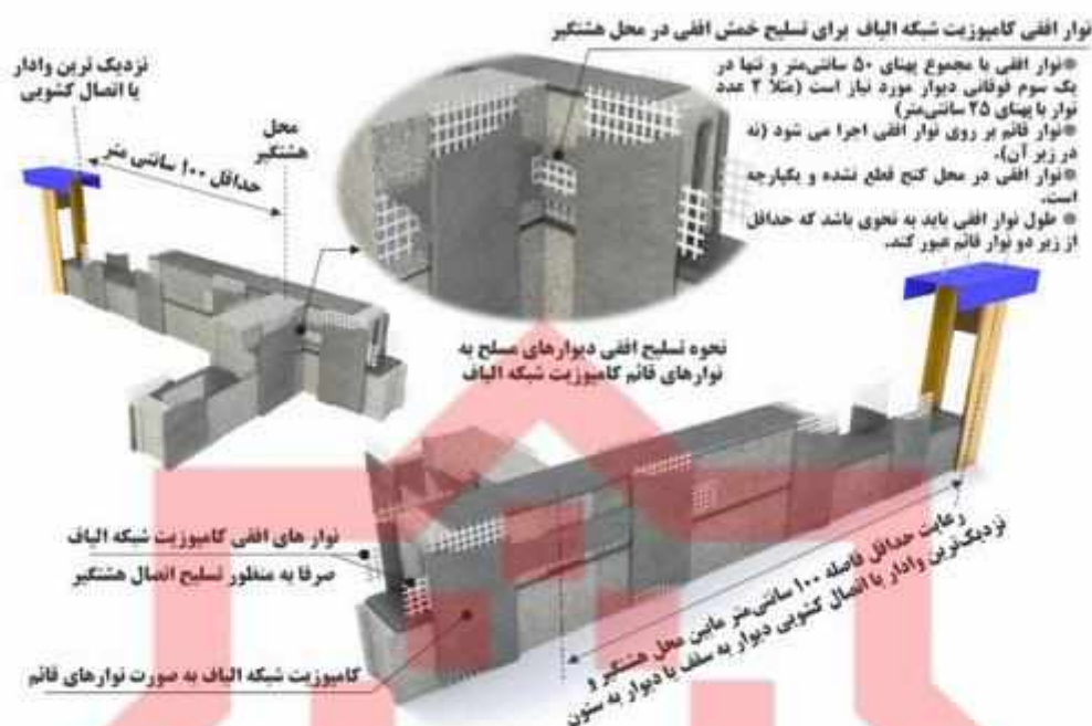
شکل ۴-۱۷ نحوه تقویت خمشی افقی در محل هسته‌گیر برای دیوارهای مسلح به نوارهای قائم کامپوزیت شبکه الیاف.
