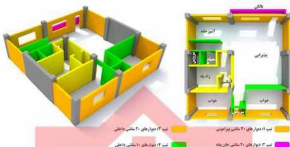
شکل ۲-۴ نمونه‌ای از تیپ بندی دیوارهای غیرسازه‌ای یک ساختمان
