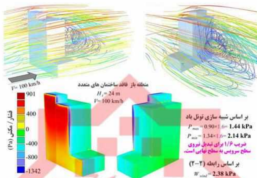
شکل پ-۱-۱ بررسی دقت رابطه (۲-۲) در تخمین فشار / مکش ناشی از باد برای یک ساختمان ۷ طبقه به ارتفاع ۲۴ متر واقع در منطقه‌ای فاقد ساختمان‌های متعدد و سرعت باد مبنای ۱۰۰ کیلومتر بر ساعت.
